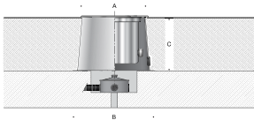
In-grade luminaire · Adjustable
